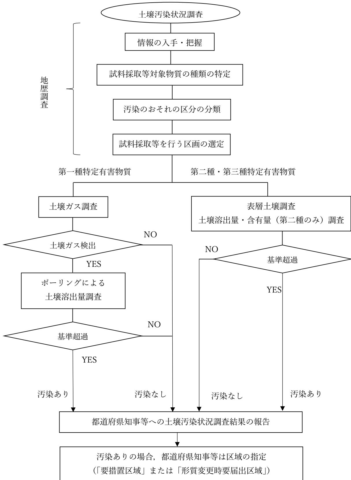
土壤汚染状況調査のフロー
